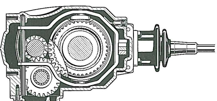
Schnitt A-B Section A-B Coupe A-B
