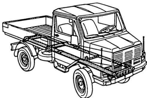
TAV. 15/2 - TELAIO PASSO 2600
