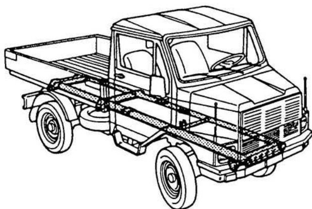
TAV. 15 - TELAIO PASSO 2600
