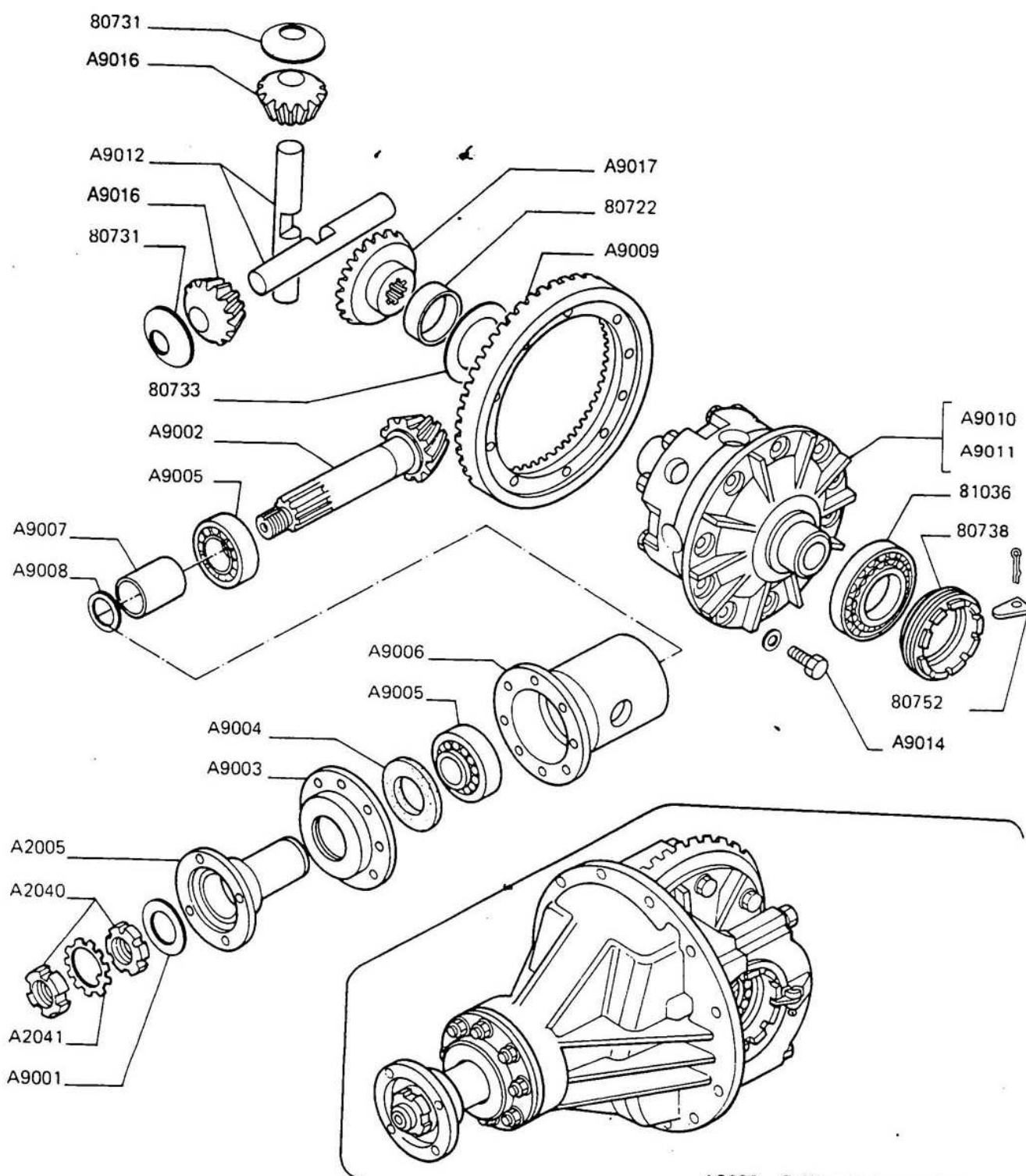
A9000 Differenziale completo posteriore
